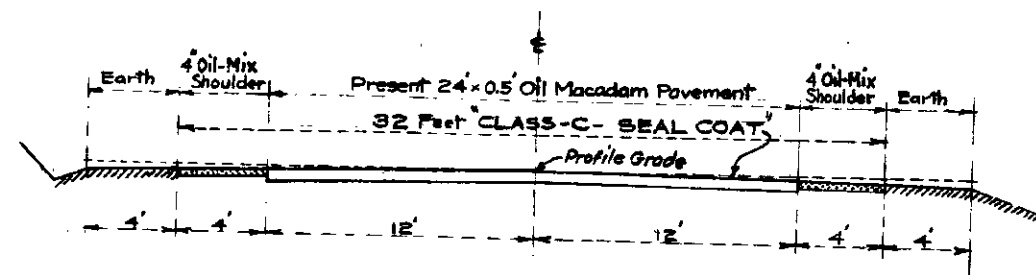
ROADWAY SECTION Scale: 1" = 4'
